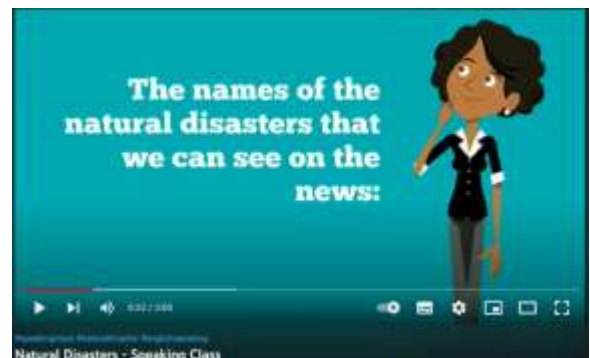
Gambar 2.tampilan aplikasi Powtoon
